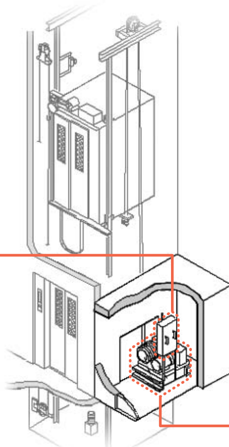
巻上機
