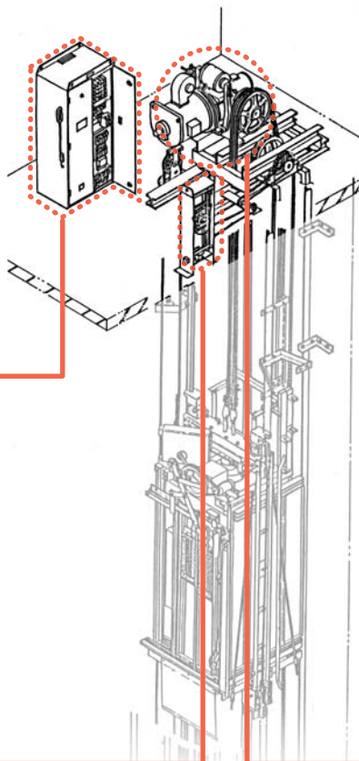
巻上機
