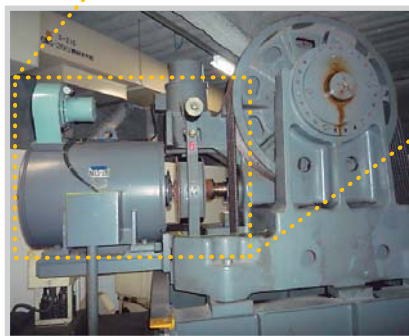
巻上機
